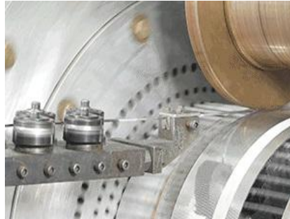
Wire rolling
